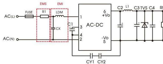
推荐电路 2
